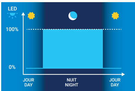
Figure 1: Profil d'éclairage durant les 3 premières nuits
