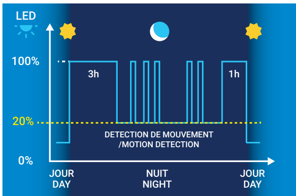
Exemple de profil d'éclairage / Example of lighting profile
